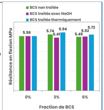
Résistance en flexion des Mortiers de bagasse de canne à sucre
