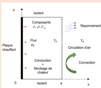
Figure 2 : Modèle physique avec ses phénomènes de transfert de chaleur dans le mur
