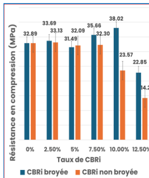
Résistance en Compression des Mortier des Cendres de Balle de Riz
