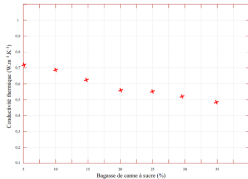
Figure 3: Conductivité thermique
