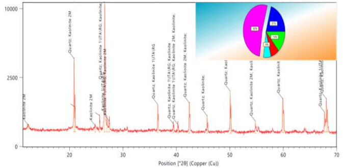
Figure 1: Diagramme de diffraction aux rayons X du composite
