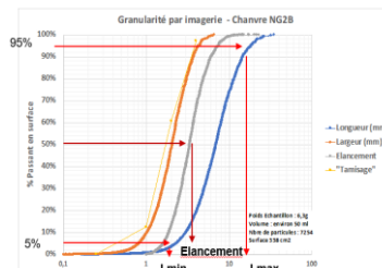
GRANULOMÉTRIE DES GRANULATS
