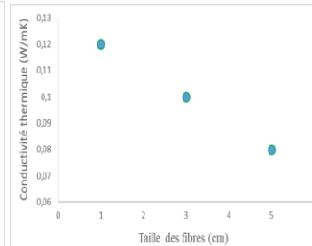
Conductivité thermique en fonction de la longueur des fibres
