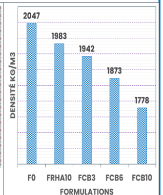
Densité des mortiers de CBRI à renfort de bagasse de canne à sucre
