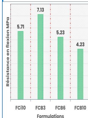
Résistance en flexion des Mortiers de CBRI à renfort de bagasse de canne à sucre
