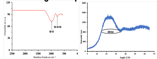
Courbe Infra-rouge
