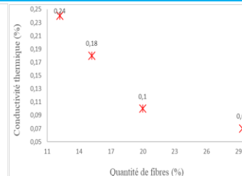
Conductivité thermique en fonction de la teneur en fibres
