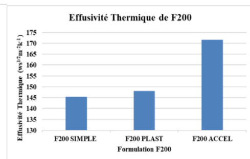
Figure 4 : Effusivité thermique
