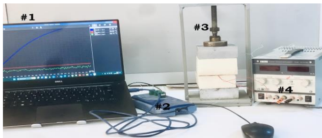
Fig-1 : Dispositif expérimental.
