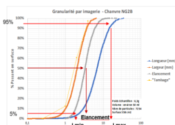
GRANULOMÉTRIE DES GRANULATS
