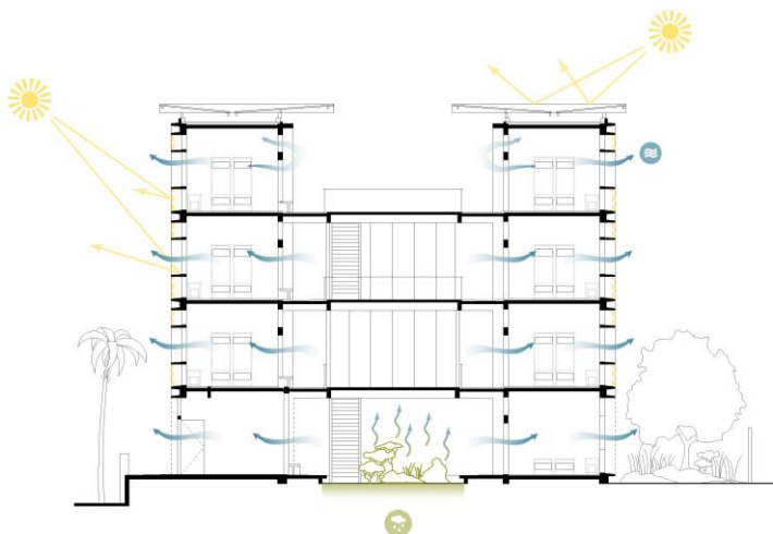
Principes bioclimatiques en coupe.
