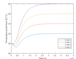
Figure 8 : Variation de la température dans CBP10 à dans l'air au cours du temps
