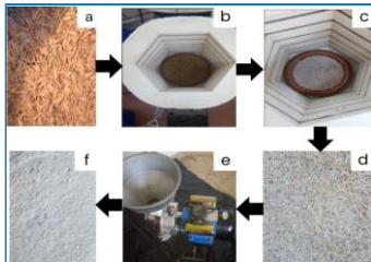
a) Balle de riz, b) balle de riz dans le four, c) cendre de balle de riz dans le four après calcination, d) cendre de balle de riz retirée du four, e) broyeur, f) cendre de balle de riz broyée.
