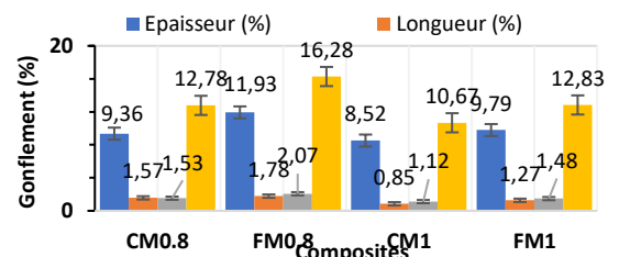
Fig. 2. Comportement des panneaux après immersion pendant 24h.
