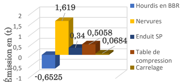
Figure 3: Diagramme des émissions par parties d'ouvrage du plancher en éco-matériaux
