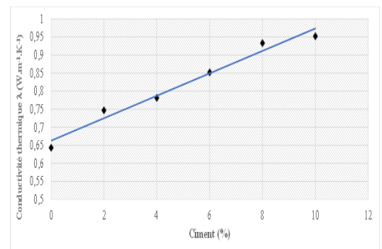
Fig. 4. Variation de la conductivité thermique des briques en terre crue en fonction de l'ajout du ciment
