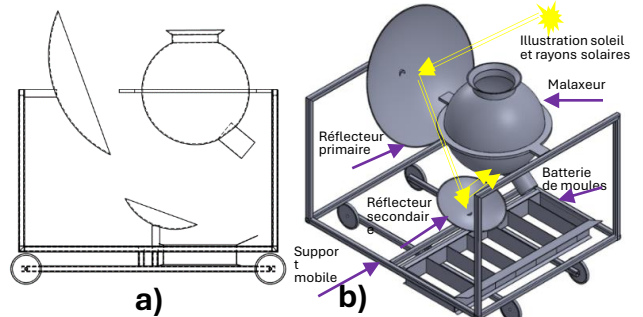
Figure 3: Dispositif de production à base d'énergie solaire a) vue de face et b) vue d'ensemble
