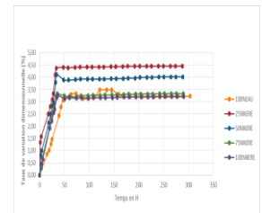
Figure 2 : Taux de variation dimensionnelle de la Terre de barre + Néré en fonction du temps..
