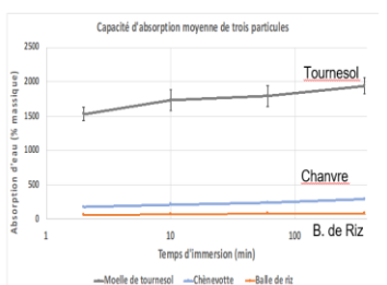
ABSORPTION D'EAU DES GRANULATS
