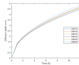
Figure 5 : Profondeur de diffusion de la chaleur au cours du temps
