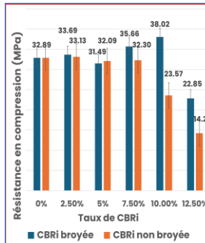
Résistance en Compression des Mortier des Cendres de Balle de Riz
