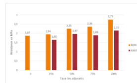
Figure 3 : Résistance en compression sur la terre de barre pour différents dosages de Néré et de karité
