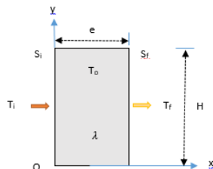
Figure 3 : Modèle physique
