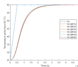
Figure 6 : Variation de la température dans les briques au cours du temps
