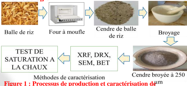
Figure 1 : Processus de production et caractérisation de la cendre
