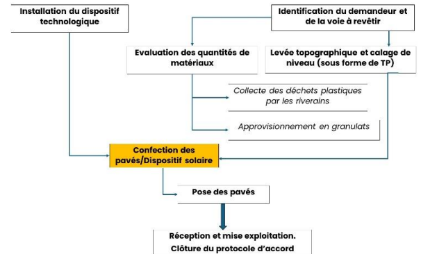
Figure 2: Synoptique de la mise en œuvre des revêtements routiers
