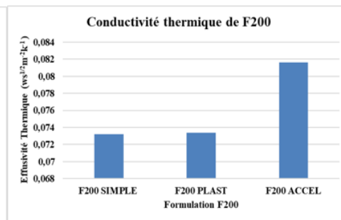
Figure 3 : conductivité thermique
