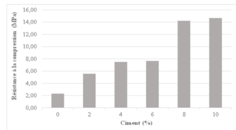
Fig. 3. Variation de la résistance à la compression des briques en terre crue en fonction de l'ajout du ciment.
