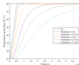
Figure 7 : Variation de la température dans CBP10 à différentes épaisseurs au cours du temps
