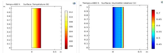
Distribution de la température à travers la paroi
