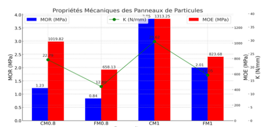
Fig. 3. Propriétés mécaniques des composites.
