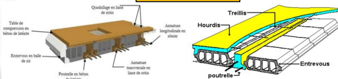
Figure 1: Schéma type de plancher en éco-matériaux
