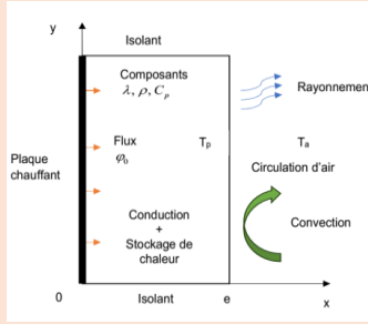
Figure 2 : Modèle physique avec es phénomènes de transfert de chaleur dans le mur
