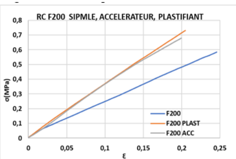
Figure 2 : Résistance à la compression en fonction du déplacement
