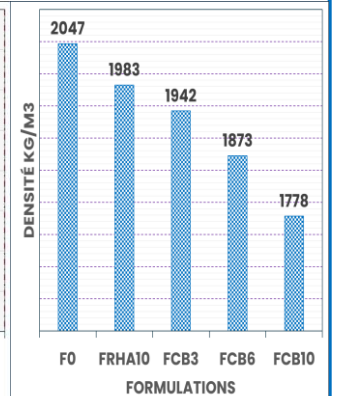
Densité des mortiers de CBRI à renfort de bagasse de canne à sucre
