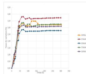
Figure 1 : Taux de variation dimensionnelle de la Terre de barre + Karité en fonction du temps.
