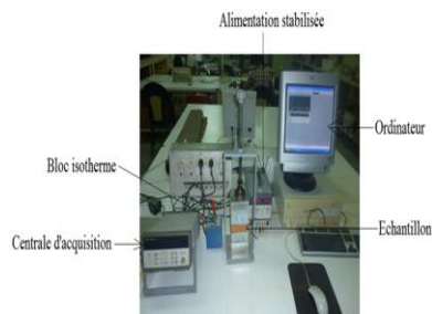
Fig. 2. Dispositif expérimental du plan chaud asymétrique
