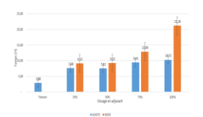
Figure 4 : Temps de résistance à la pénétration pour différents taux de stabilisants organiques.
